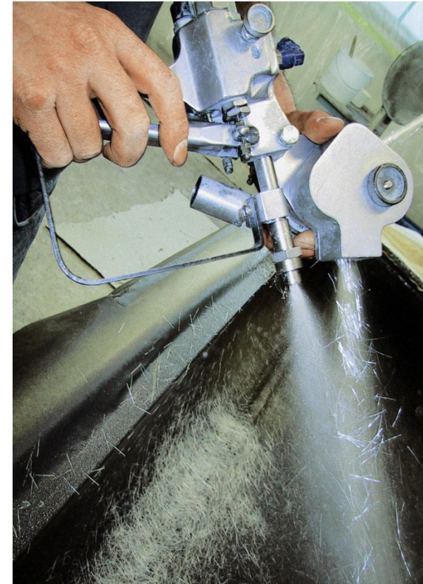
Szálszóró pisztoly
