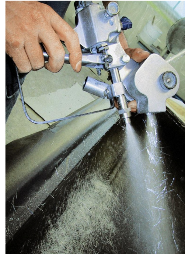
Szálszóró pisztoly
